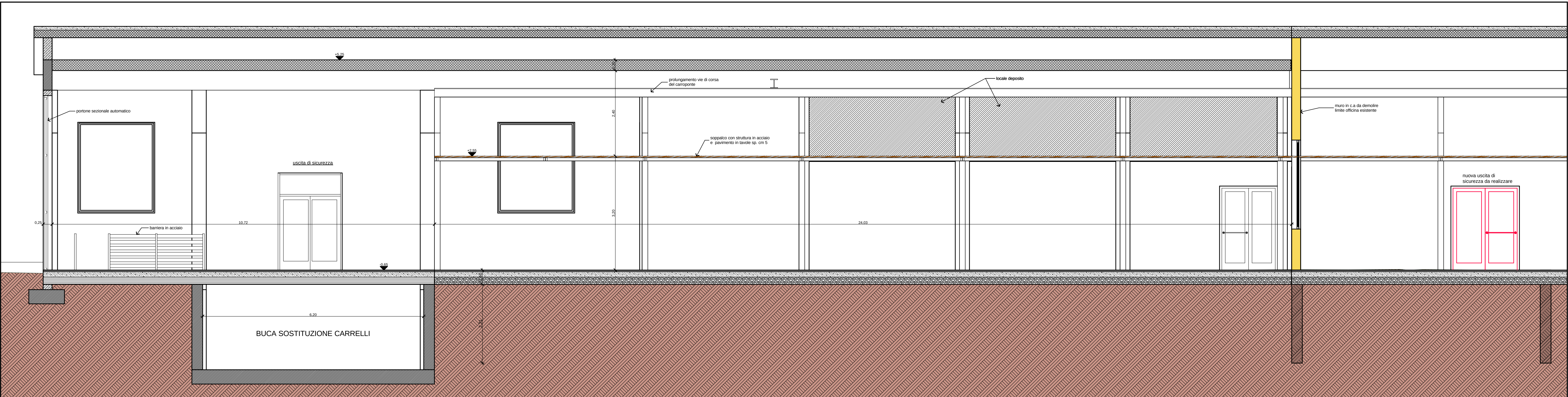
SEZIONE D2
