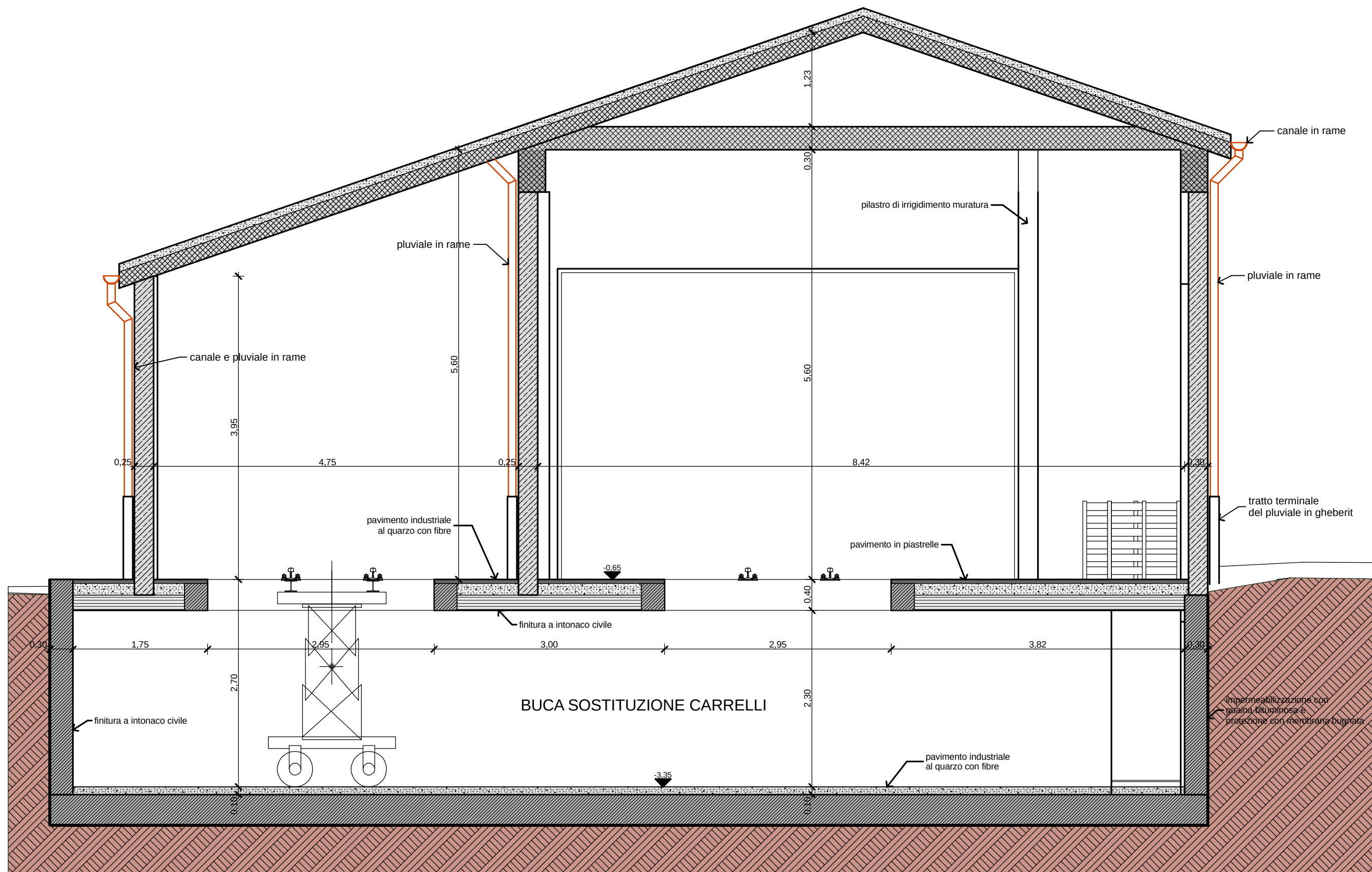
SEZIONE D/1
