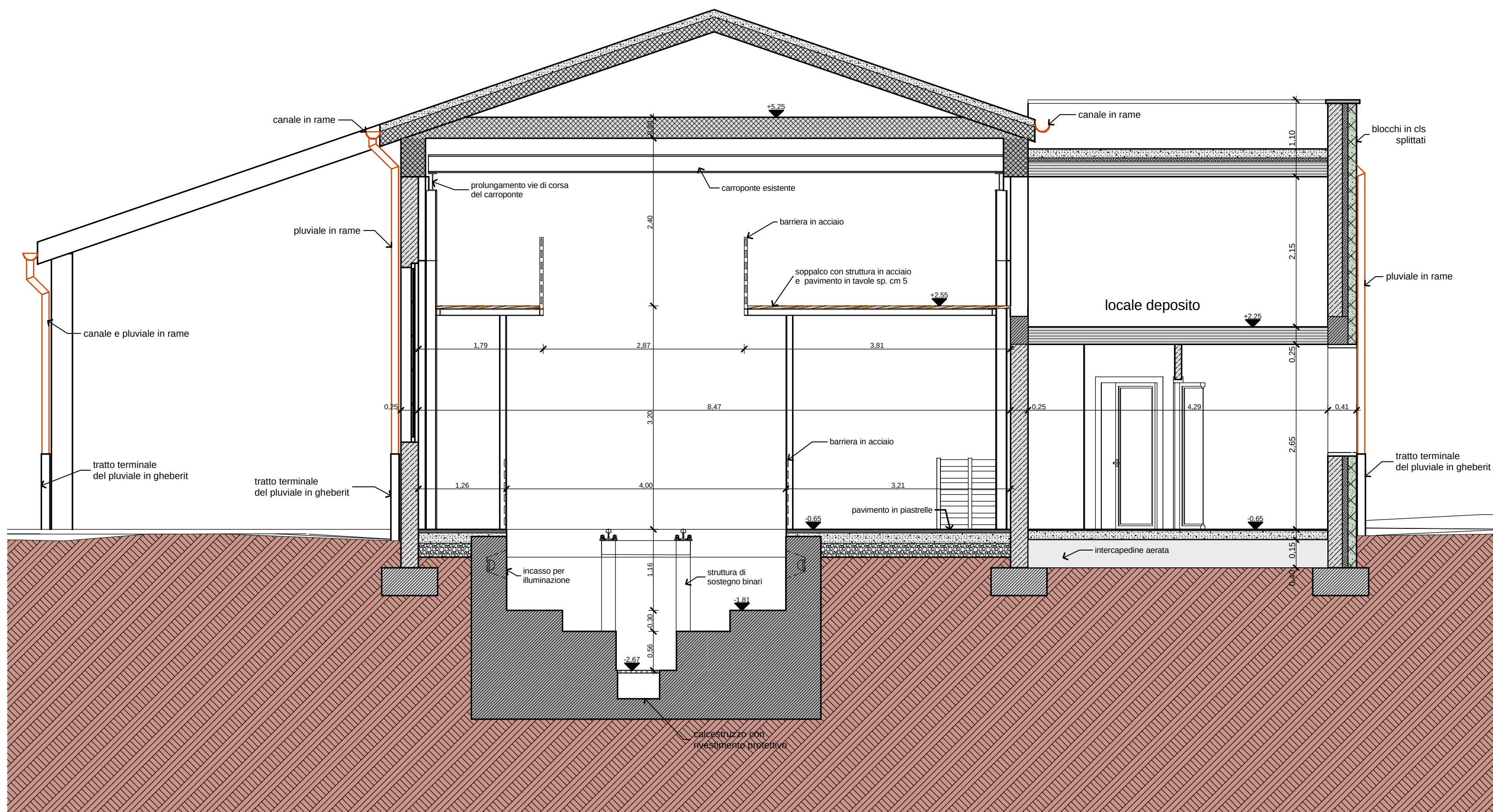
SEZIONE D/1
