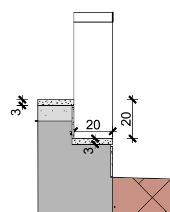
SEZIONE S2 scala 1/20
